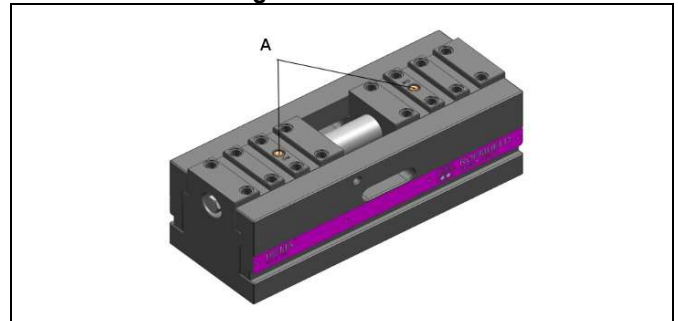
Fig. 3 : Lubrification de la broche par graisseur (A) pour type 100 + 125
