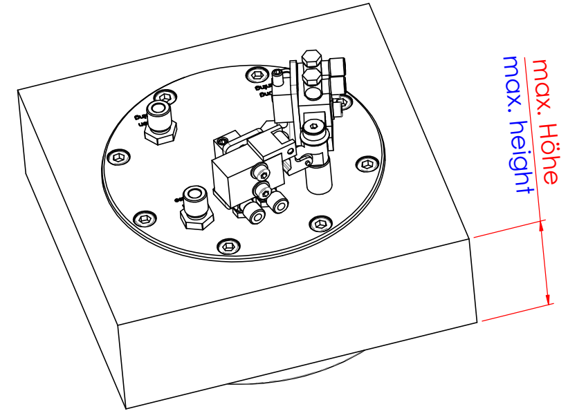
Einbaubeispiel 1 installation example 1
