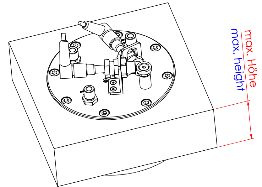
Einbaubeispiel 2 installation example 2
