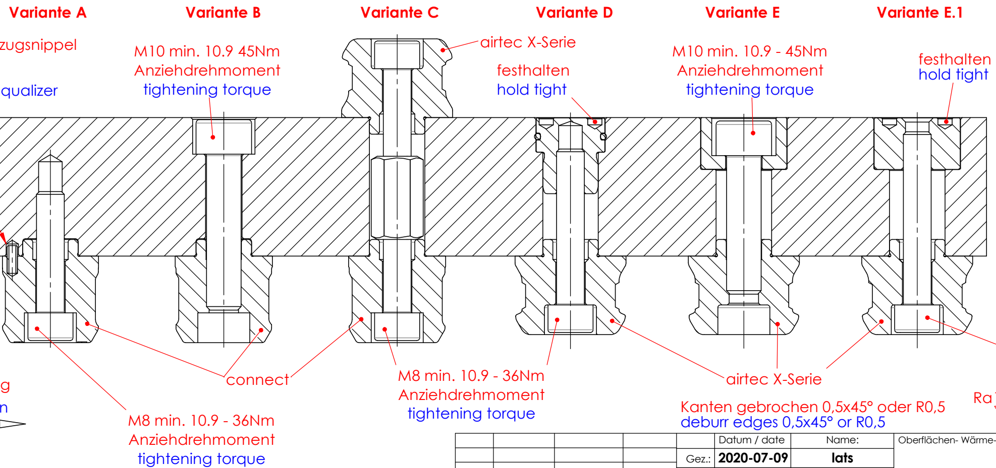
Einbaumaße/Beispiele gelten für alle STARK.connect & STARK.airtec X-Serie Einzugsnippel assembly dimensions/examples apply for all STARK.connect & STARK.airtec X-Serie retractable nipple
